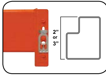
STEP LOAD BEAMS
