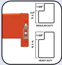
STEP LOAD BEAMS
